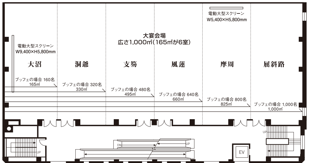
20.2m×48.5m 天井高6.3m
