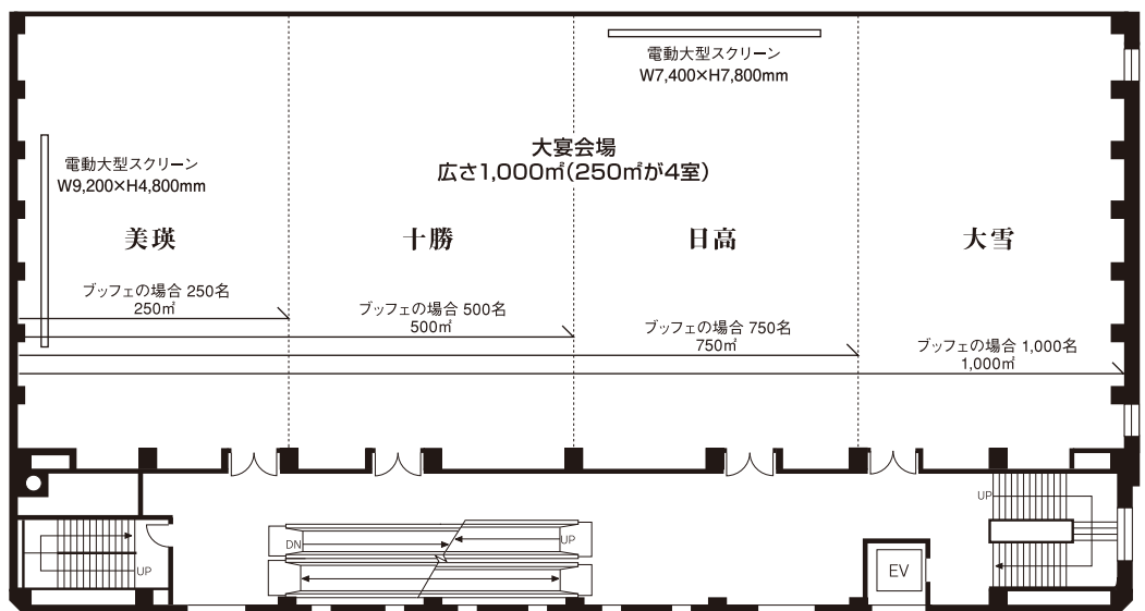
20.2m×48.5m 天井高8.3m
